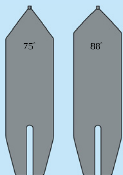
切領針座 Collar trimming template (75°、88°)
