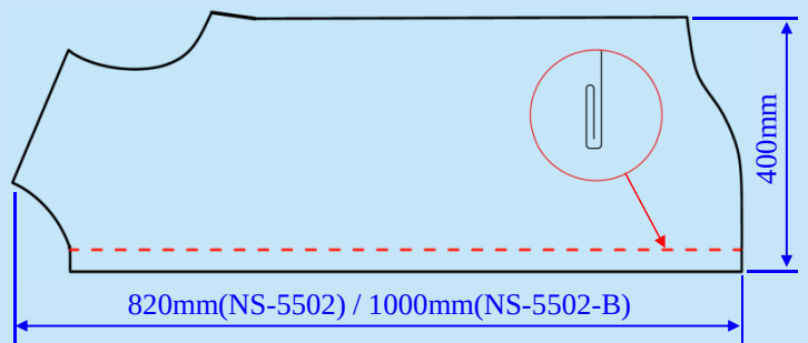
最大折前幅裁片尺寸 Max. foldable placket size
