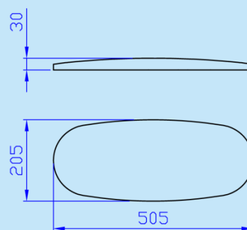
最大下模尺寸圖 Max. lower Mould Dimensions
