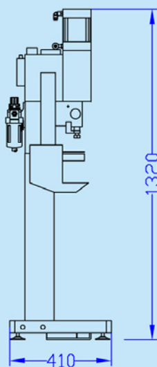
機身外形尺寸圖 Machine Outline Dimensions Diagram
