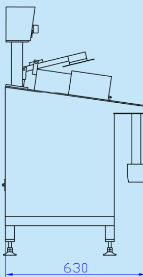
NS-9082-N 機身外形尺寸圖 Machine external dimensions diagram
