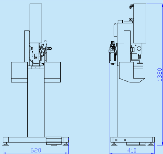
機身外形尺寸圖 Machine Outline Dimensions Diagram
