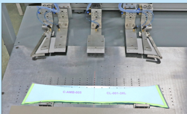
立體領操作 3D collar run-stitch operation
