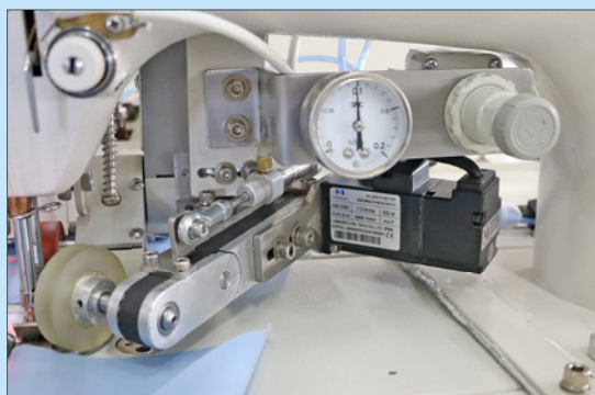
自動撥布裝置 Automatic fabric spreading device
