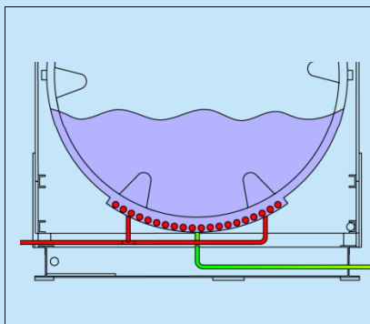
O-I-63-05 / O-I-63-07 間接保溫系統-內部 Indirect insulation system-Internal
