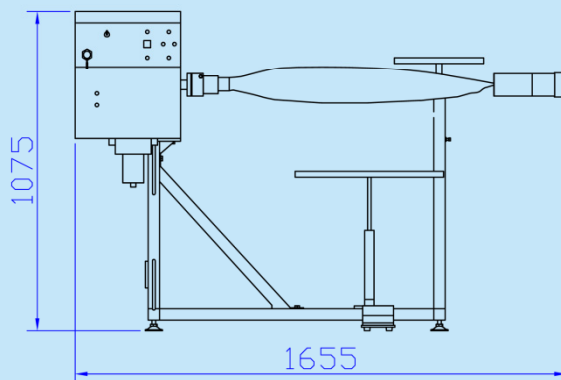
機身外形圖Machine Size (Unit : mm)
