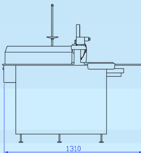
機身外形尺寸圖 Machine external dimensions diagram
