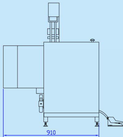
機身外形尺寸圖 Machine external dimensions diagram
