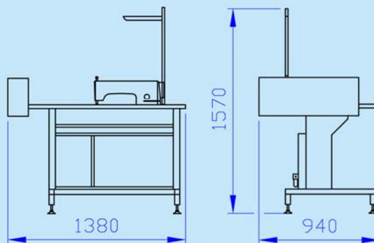
機身尺寸 Machine size
