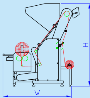
機器外形圖:Machine Size (mm)
