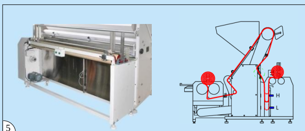
自動鬆布系統 Automatic Fabric Loosening System
