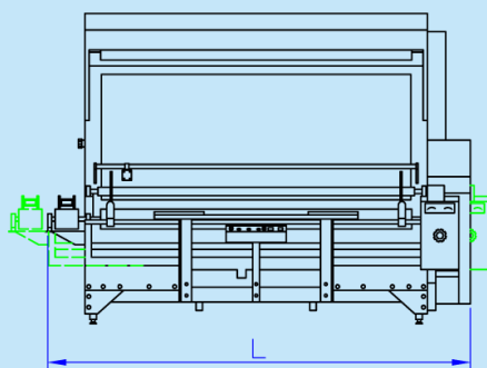
機器外形圖:Machine Size (mm)
