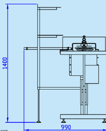
外形尺寸圖 Overall Size Diagram
