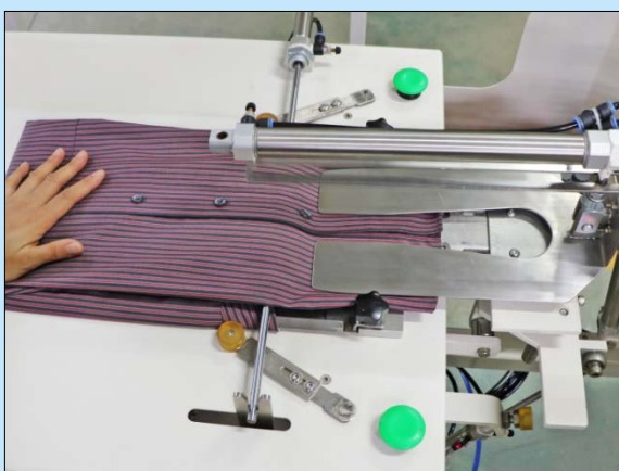
自動摺衫推板裝置，可將衫腳自動插入 Tuck-in device can automatically push shirt bottom inside
