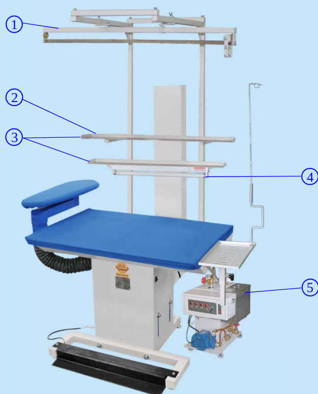
NS-3520 ~ NS-3523 系列熨檯 NS-3520 ~ NS-3523 Series Ironing Table
