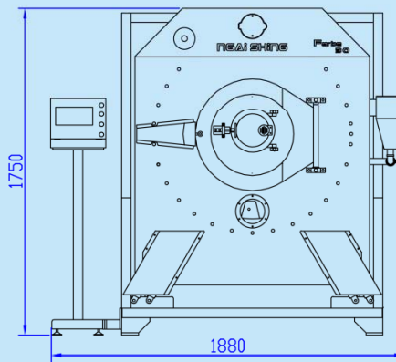
機身尺寸簡圖(單位：mm) Machine size diagram(unit: mm)
