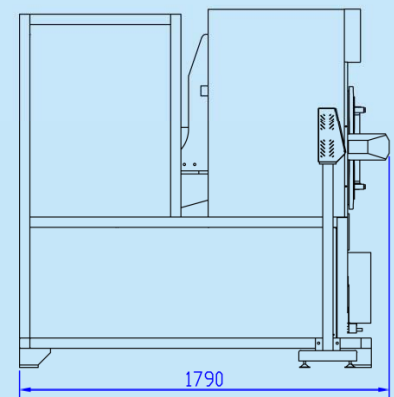
機身尺寸簡圖(單位：mm) Machine size diagram(unit: mm)
