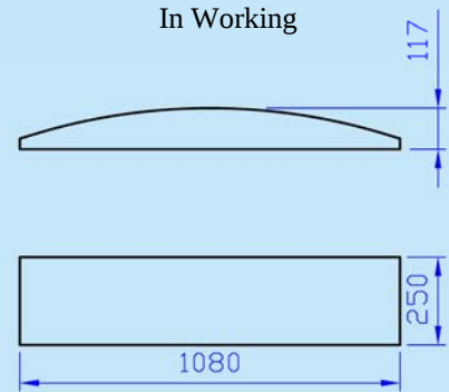
下模尺寸簡圖 Lower Mould Dimensions
