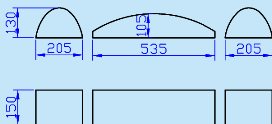
NS-9243M 下模尺寸圖 Lower mould dimension diagram
