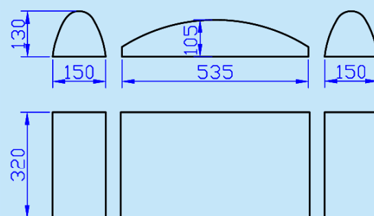
NS-9243F-L 下模尺寸圖 Lower mould dimension diagram
