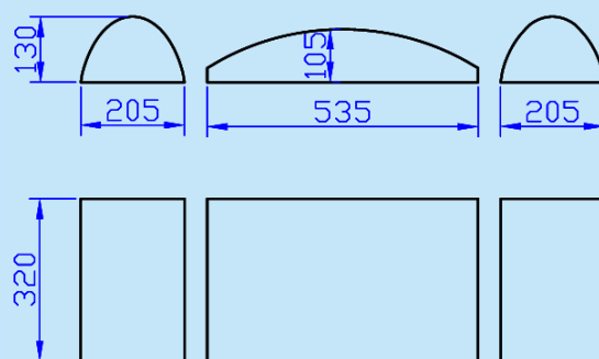
NS-9243M-L 下模尺寸圖 Lower mould dimension diagram
