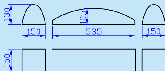
NS-9243F 下模尺寸圖 Lower mould dimension diagram
