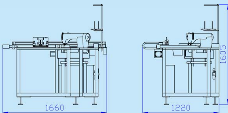
機身尺寸簡圖(單位:mm) Machine size diagram (unit: mm)
