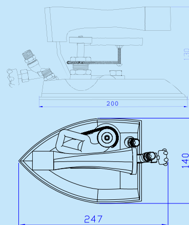
熨鬥尺寸簡圖 Iron Dimensions Diagram (mm)
