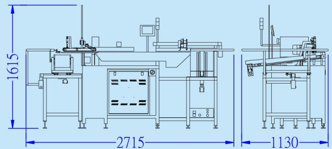
機身尺寸圖 Machine Size(mm)
